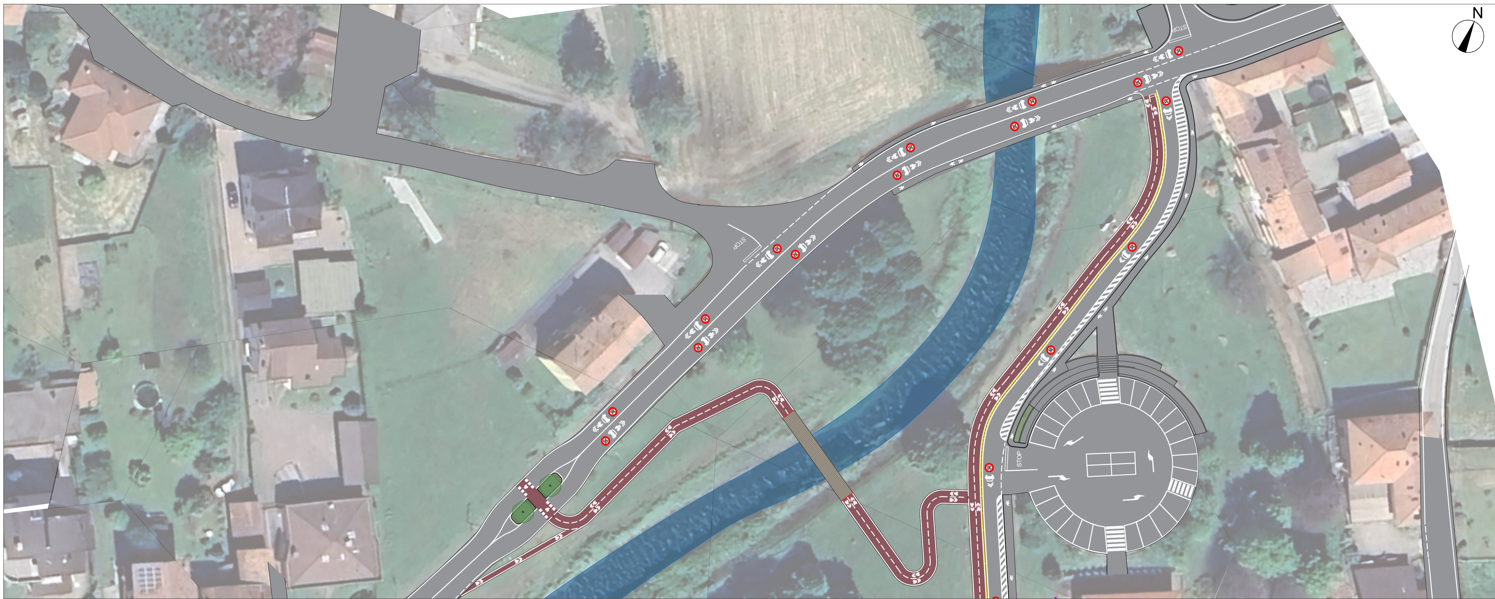
STATO DI PROGETTO Scala 1:500
