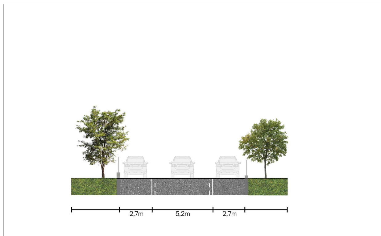
STATO DI FATTO Sez.08 - 1:200
