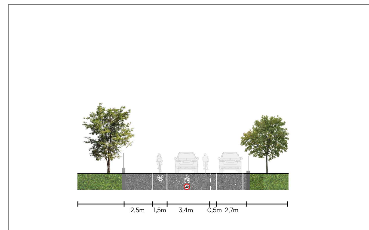
STATO DI PROGETTO Sez.08 - 1:200
