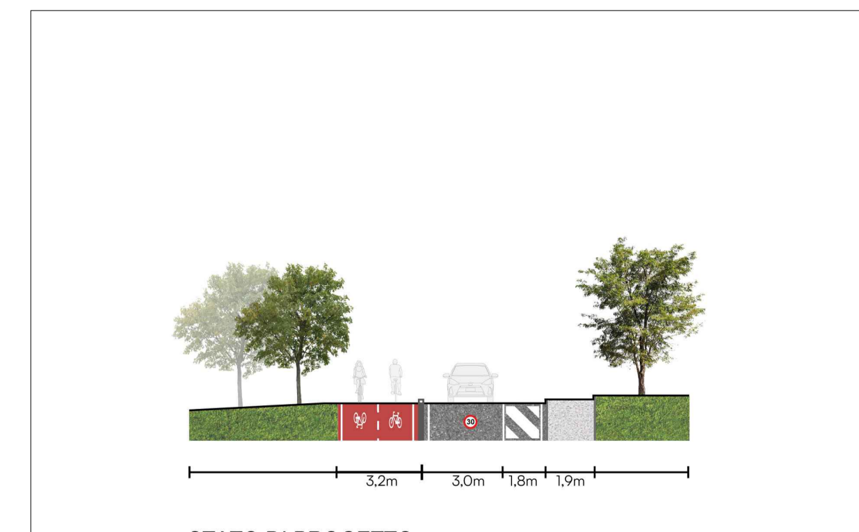
STATO DI PROGETTO Sez.09 - 1:200
