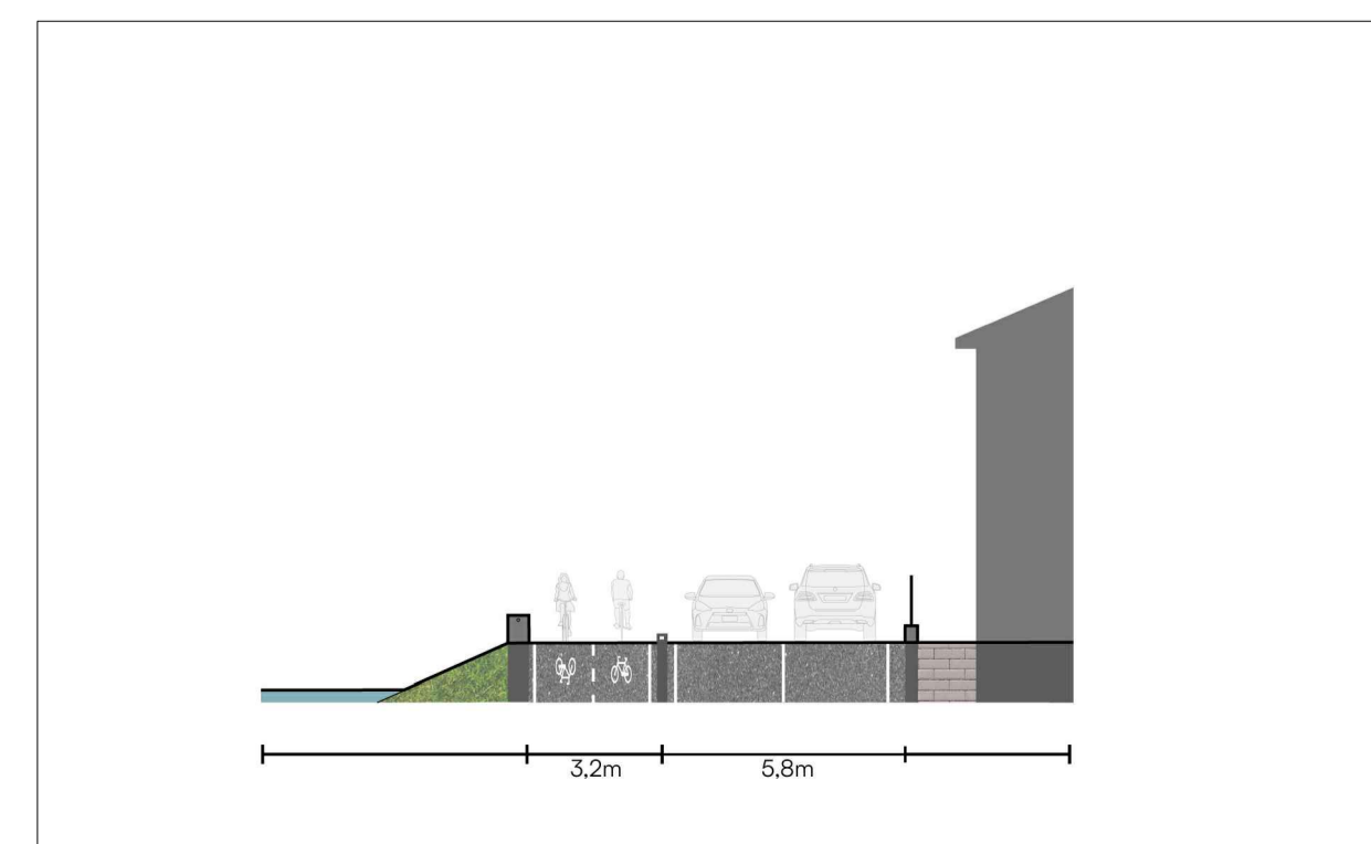
STATO DI PROGETTO Sez.01 - 1:200
