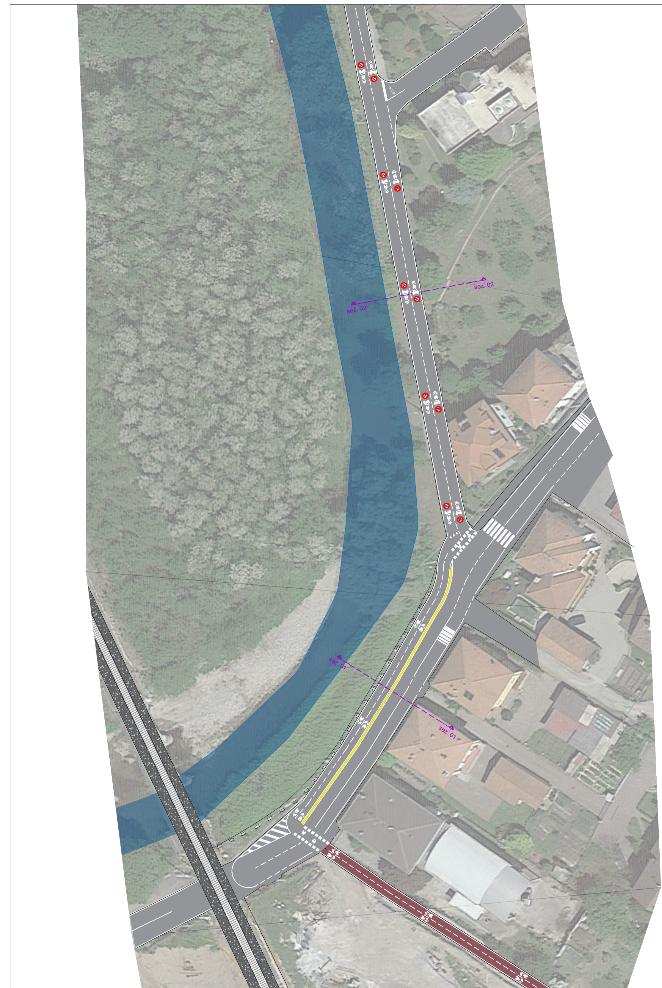
STATO DI PROGETTO Scala 1:500
